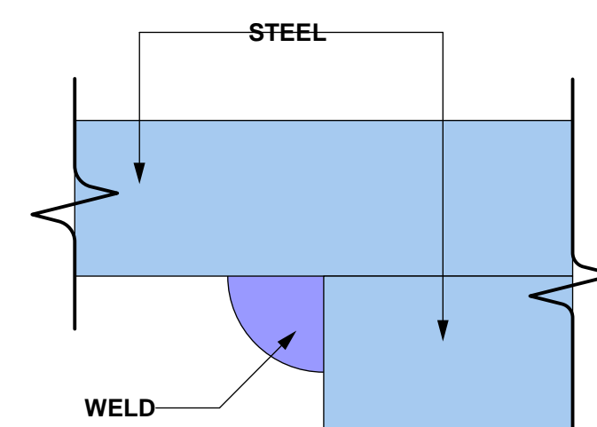
FILLET WELD
